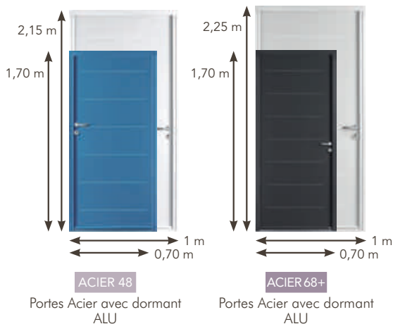
ÉQUATION HAUTEUR MAXIMUM AVEC IMPOSTE H 2350 L 900 Au-delà de 2250 mm, possibilité de mettre une imposte de 200 à 450 mm pour une hauteur maximum porte + imposte de 2350 mm.
